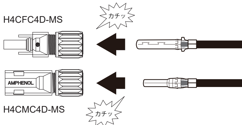
図 5-5 正極および負極コネクタの挿入
