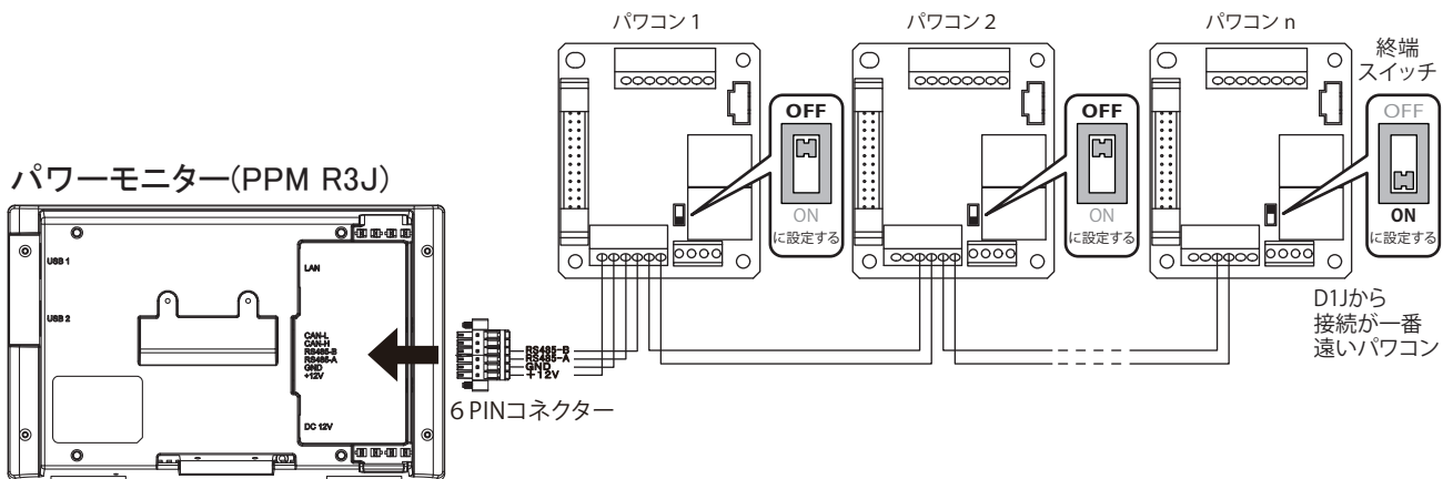
図 5-11 複数のパワーコンディショナを接続するとき
