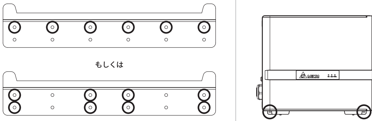
図 4-2 壁への正しいネジ位置のイメージ図
