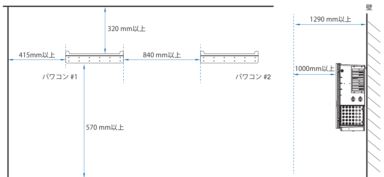
図 4-3 マウントベースとネジ穴のイメージ図
