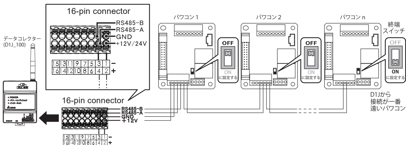
図 5-9 複数のパワーコンディショナを接続するとき
