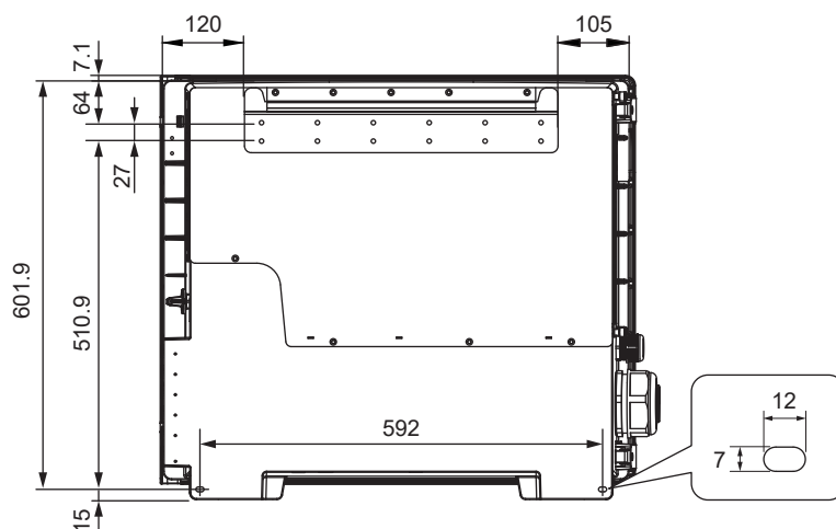
図 4-1-a マウントベースと本体背面図
