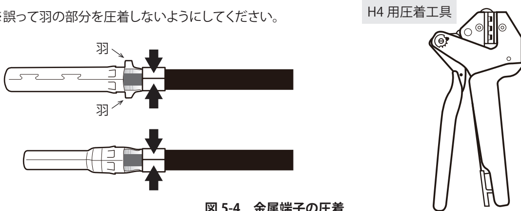
図 5-4 金属端子の圧着
