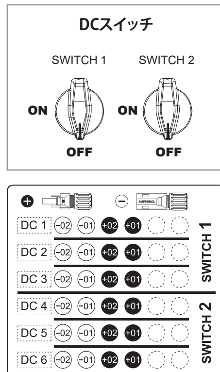
図8-1 DCスイッチのON/OFF
