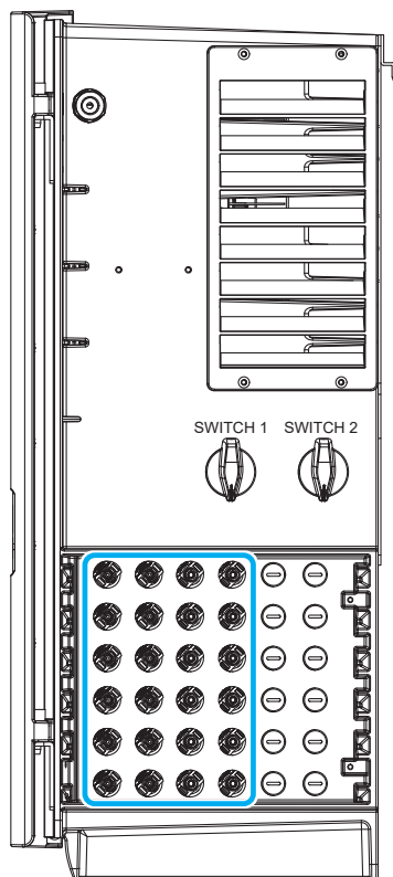
図8-1 DCスイッチのON/OFF
