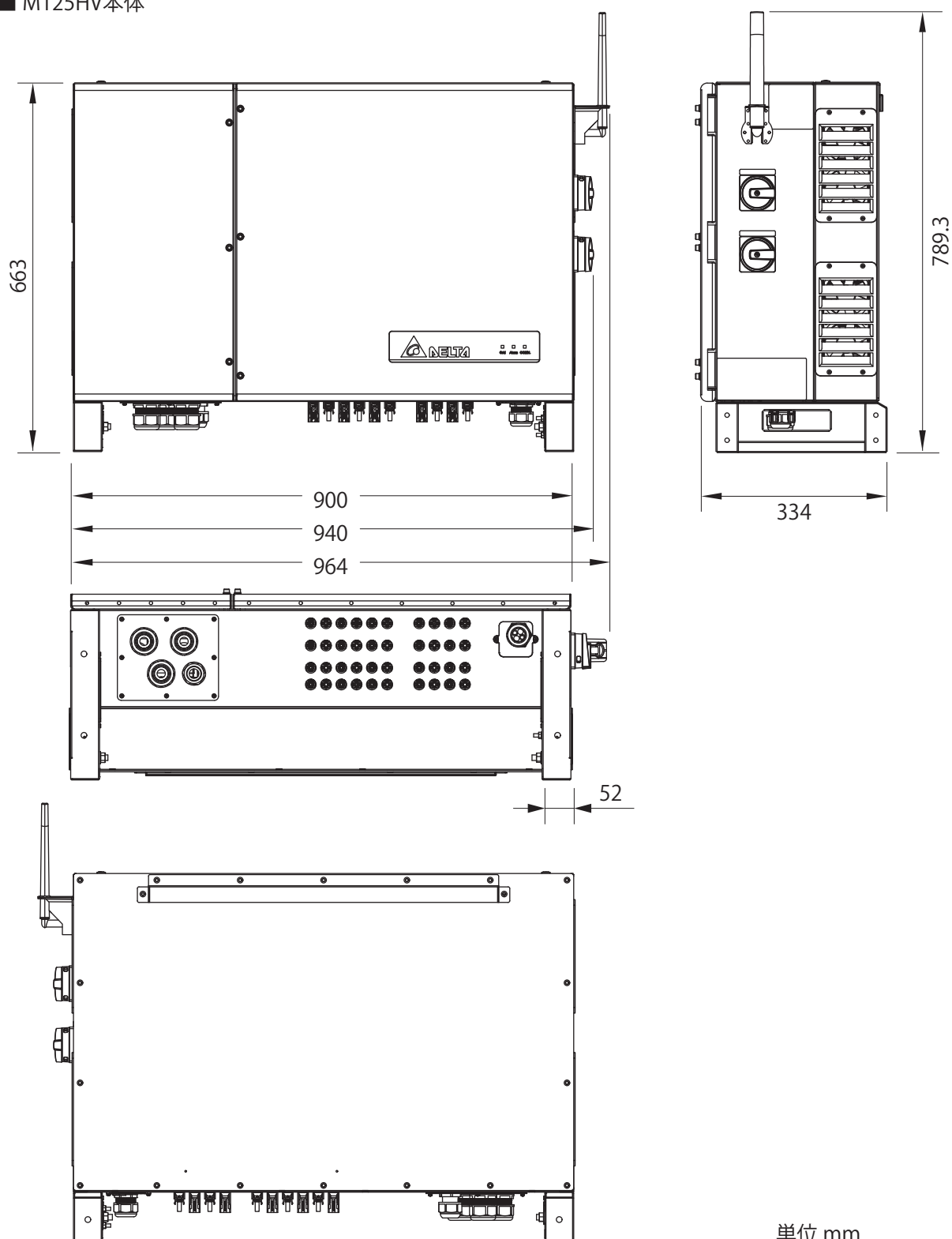
図 3-1 M125HV 本体寸法図
