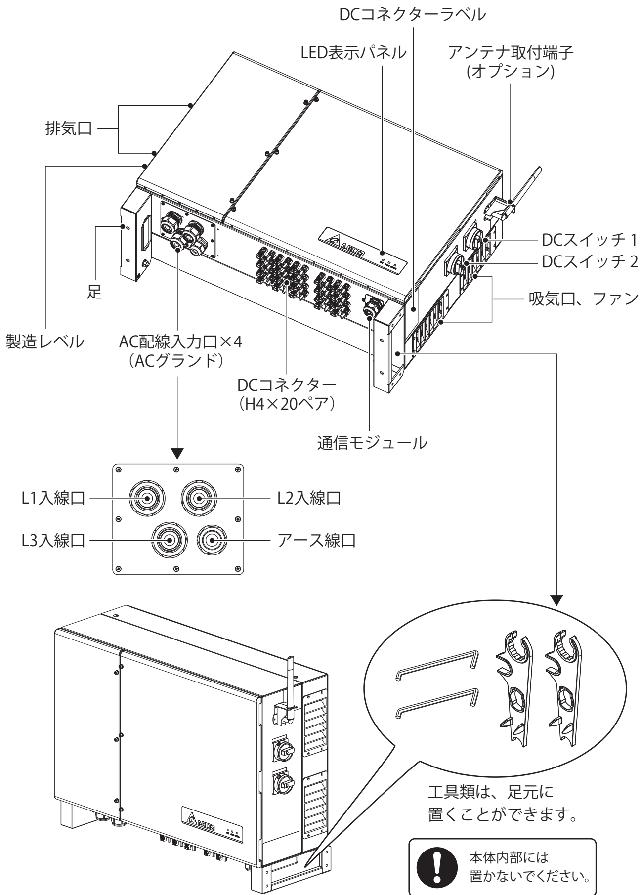
図 3-4 各部の名称
