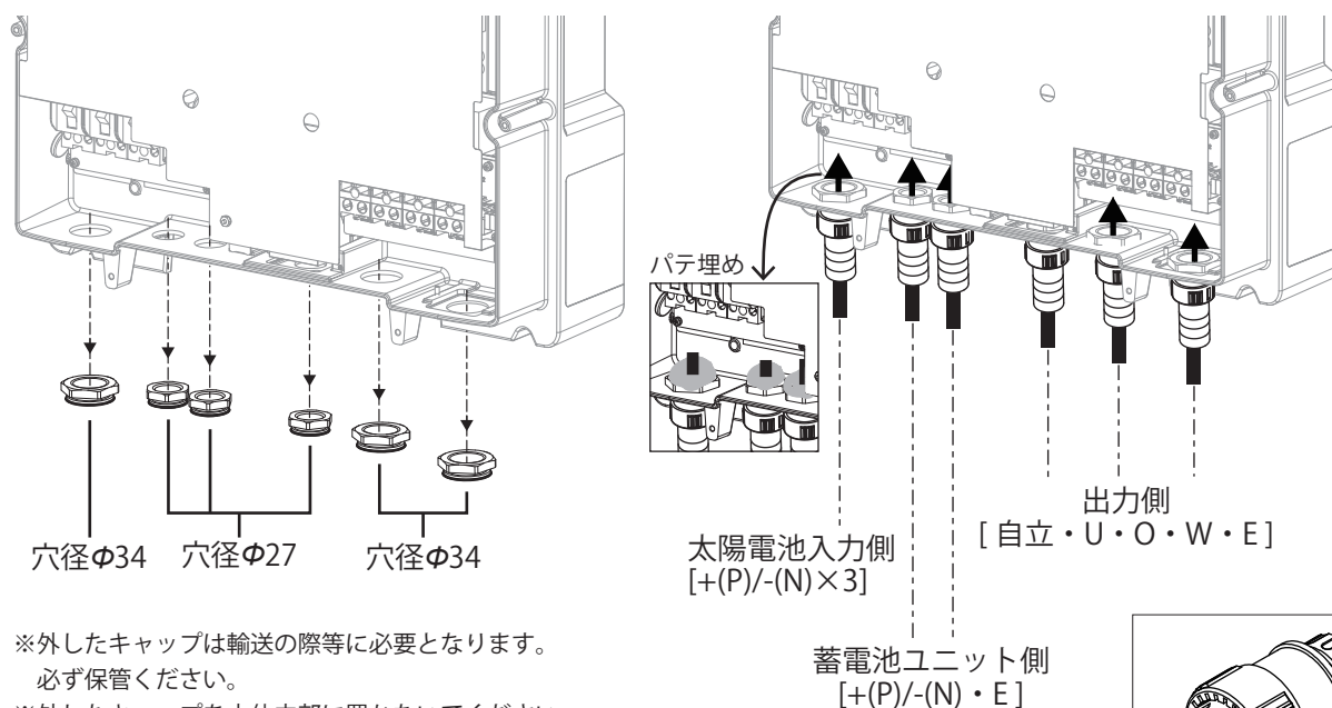
PF 管用コネクター (防水型)
